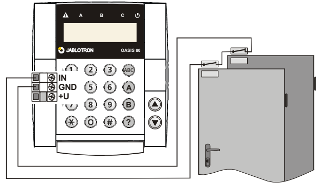
Példa az ajtónyitás érzékelő bekötésére.
